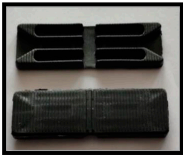
Taco para base de vidrio (80*28*4) mm
