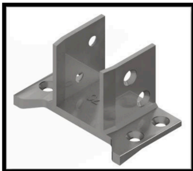
Conector travesaño 642
