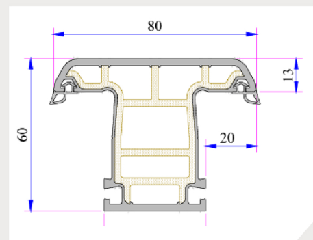
Perfil División
