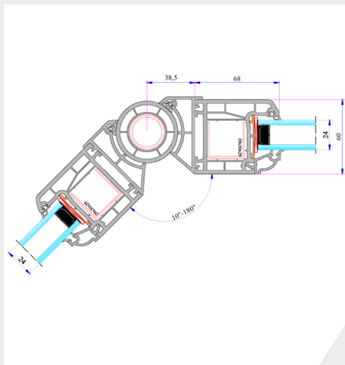
Ventana con perfil circular 10° a 180°
