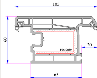
Perfil Hoja Puerta Exterior
