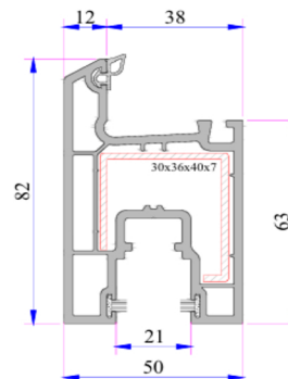
Perfil Hoja
