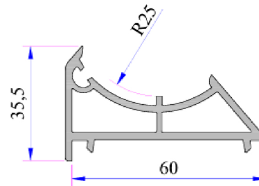
Adaptador de Perfil Circular
