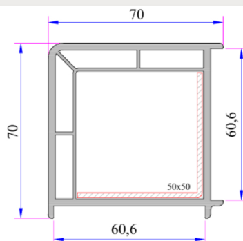
Perfil para Esquina 90°
