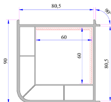
Perfil para Esquina 90°
