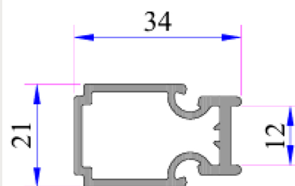
Adaptador de hojas (Aluminio)
