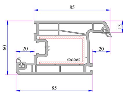
Perfil Hoja Puerta Interior
