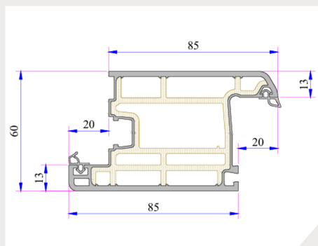
Perfil Hoja Puerta Interior
