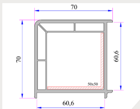
Perfil para Esquina 90°
