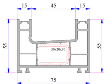
Perfil Marco Doble Riel
