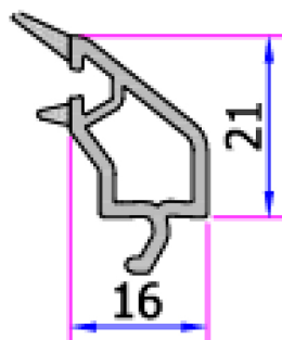
Sujetador de Vidrio 24 mm
