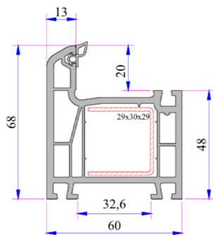
Perfil Marco
