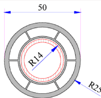
Perfil Circular
