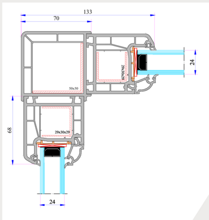
Ventana con perfil esquina cuadrado 90°
