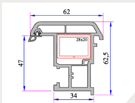
Travesaño móvil
