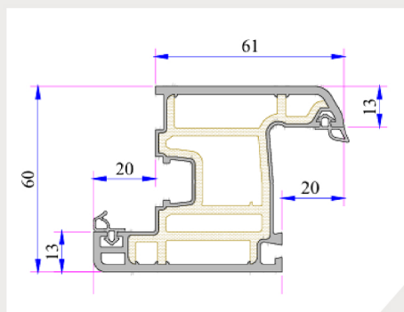
Perfil Hoja
