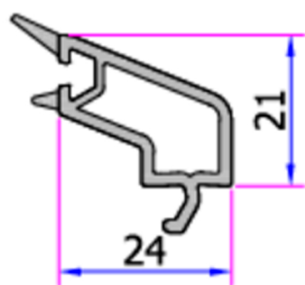
Sujetador de Vidrio 8
