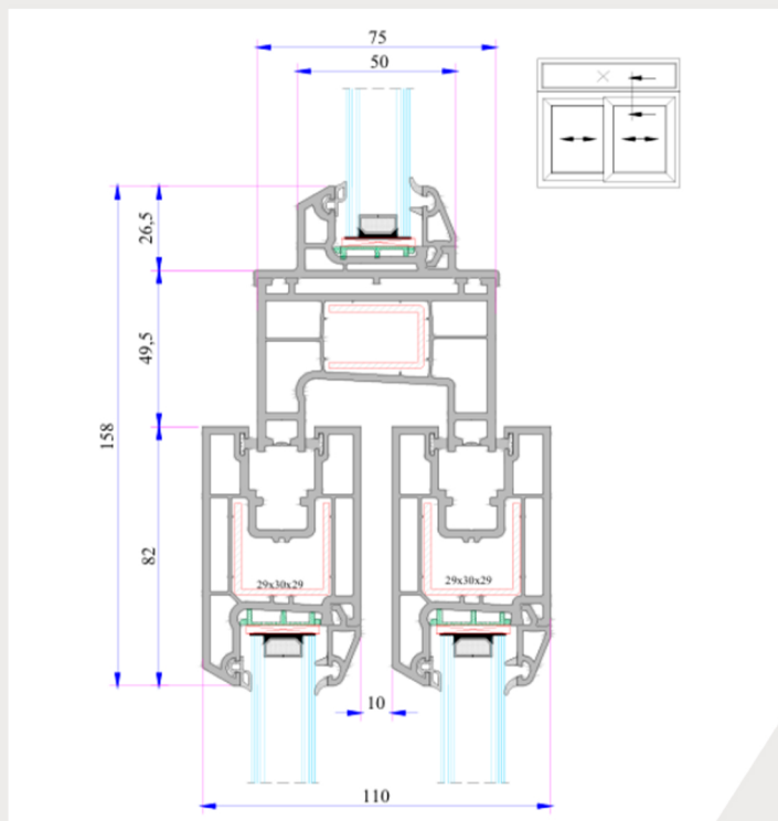
Ventana corrediza con fijo superior
