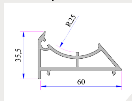
Adaptador de Perfil Circular
