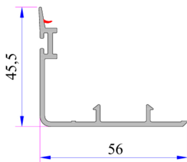
Cubierta de Perfil de Hoja
