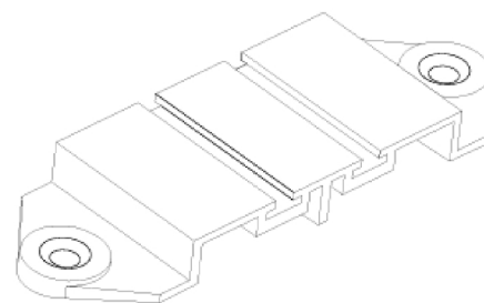
Corta Viento
