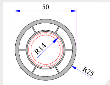
Perfil Circular
