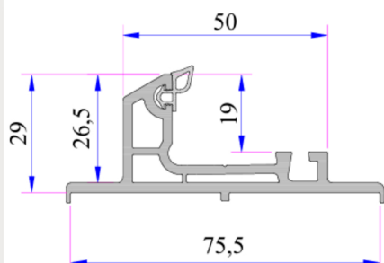
Perfil Adaptador de Fijo
