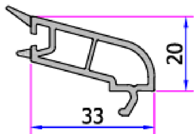
Sujetador de Vidrio 6 – 8 mm
