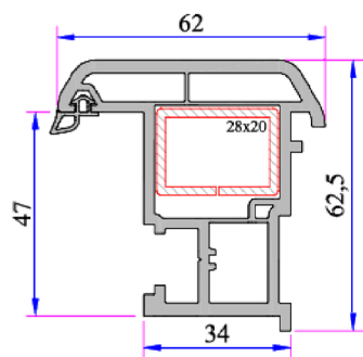
Travesaño móvil
