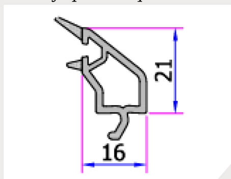
Sujetador de Vidrio 24 mm
