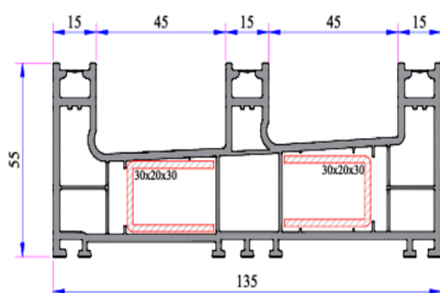
Perfil Marco Triple Riel
