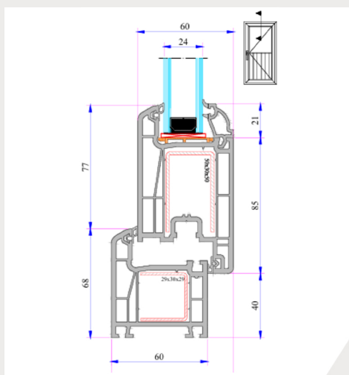
Puerta Apertura Interior
