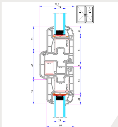
Ventana con travesaño móvil
