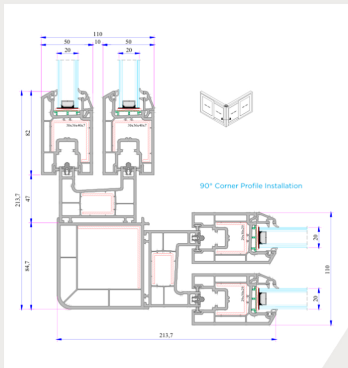
Ventana en esquina 90°
