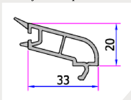
Sujetador de Vidrio 6 – 8 mm
