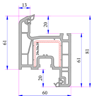
Perfil Hoja
