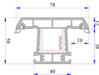
Perfil Divisor
