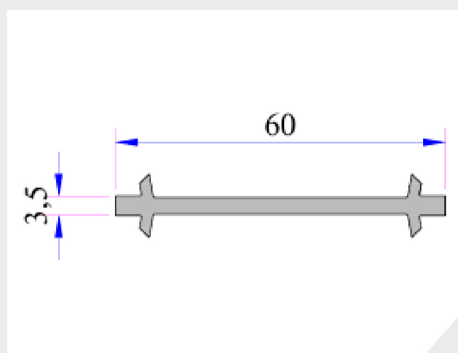
Perfil de Acoplamiento
