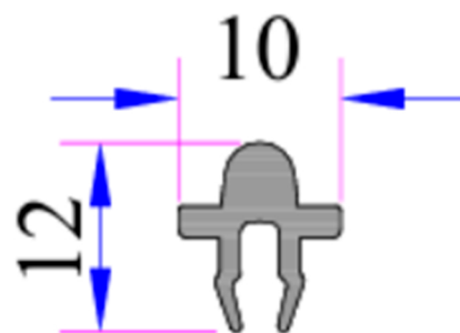
Riel (Aluminio)
