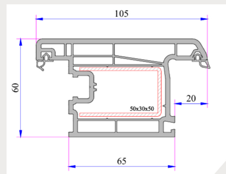
Perfil Hoja Puerta Exterior
