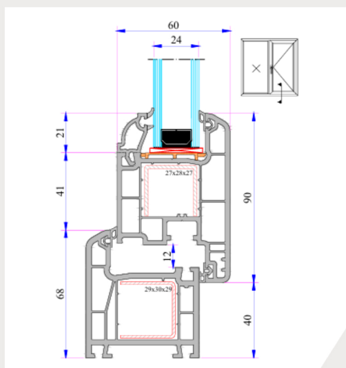
Ventana Exterior
