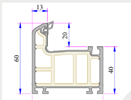
Perfil Marco
