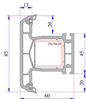
Perfil División
