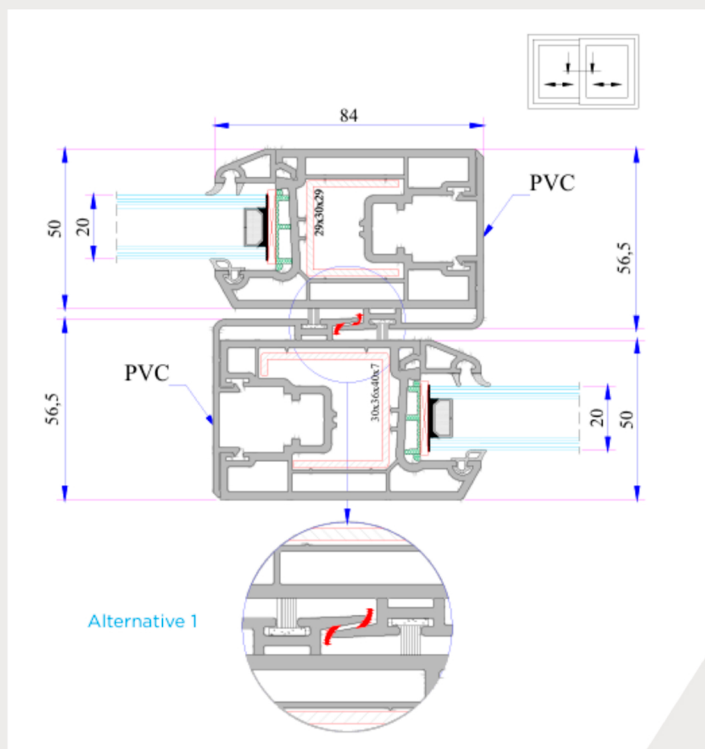
Instalación de cubierta de hojas (TRASLAPE)
