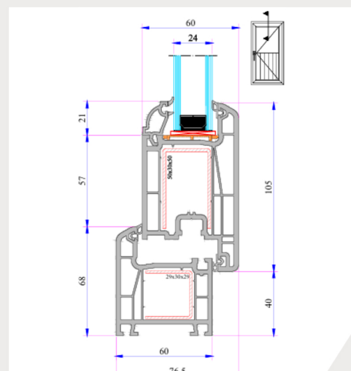
Puerta Apertura Exterior
